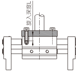
轴向螺纹孔安装
