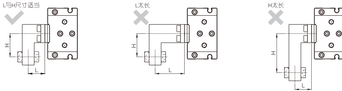
闭合夹持点范围
