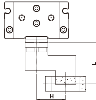
张开夹持点范围
