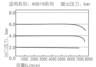
高压型流量特性
