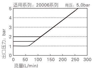
中压型溢流特性
