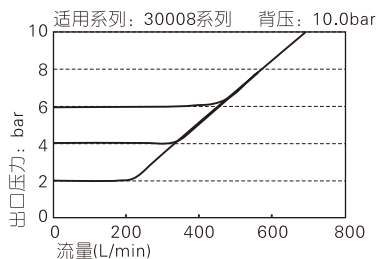
高压型溢流特性
