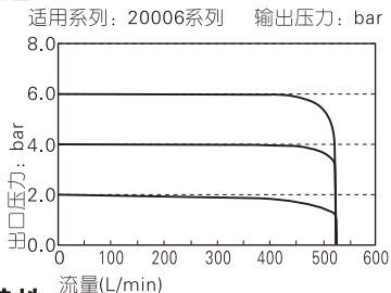
高压型流量特性
