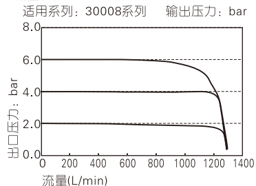
高压型流量特性
