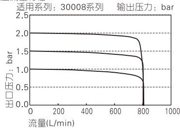
中压型流量特性
