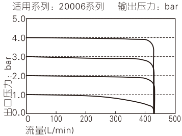
高压型流量特性
