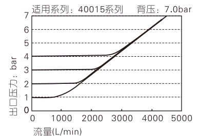
高压型溢流特性
