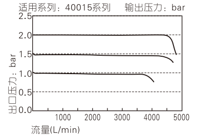
中压型流量特性
