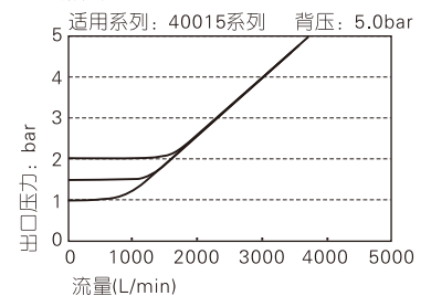
中压型溢流特性
