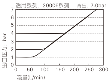
高压型溢流特性
