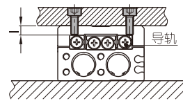
顶板安装
